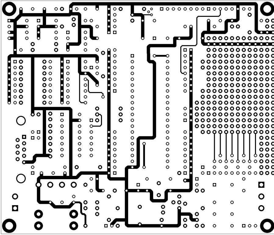
“TOP LAYER” dimensioni reali
