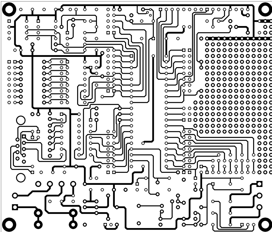
“BOTTOM LAYER” visto in trasparenza dal TOP dimensioni reali
